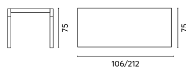
Art. RTA 40B TAVOLO CAPANNORI 106/212 cm Tavolo allungabile da balcone Piano a doghe in alluminio
