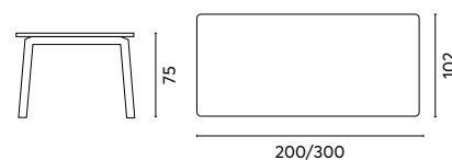
Art. RTA 63G TAVOLO PORTO ERCOLE 200/300 cm Piano in alluminio Allungo centrale
