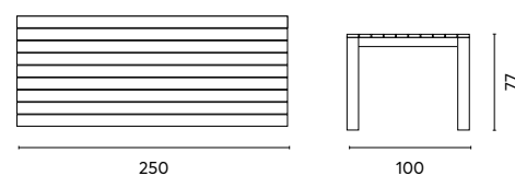
Art. WRT 06 TAVOLO GIACARTA
