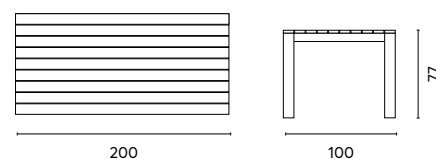
Art. WRT 01 TAVOLO GIACARTA
