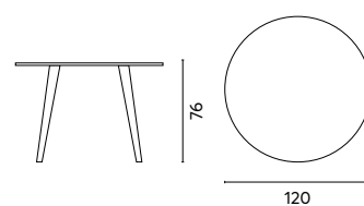
Art. RTA 22G TAVOLO ALBERESE ROTONDO Ø 120 cm Piano in alluminio
